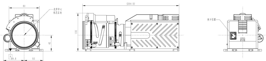
网口 25~75mm 变焦版
